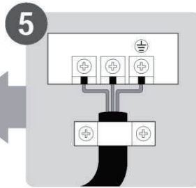
Kabloları bağlayın
