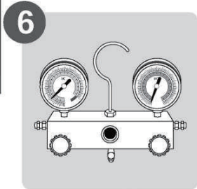
Soğutucu sistemini tahliye edin
