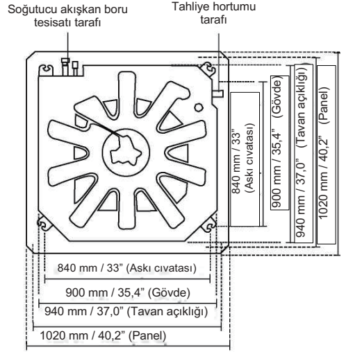
60 K Süper İnce modellerin tavan delik boyutu
