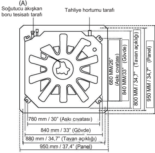
18-48 K Süper İnce modellerin tavan delik boyutu
